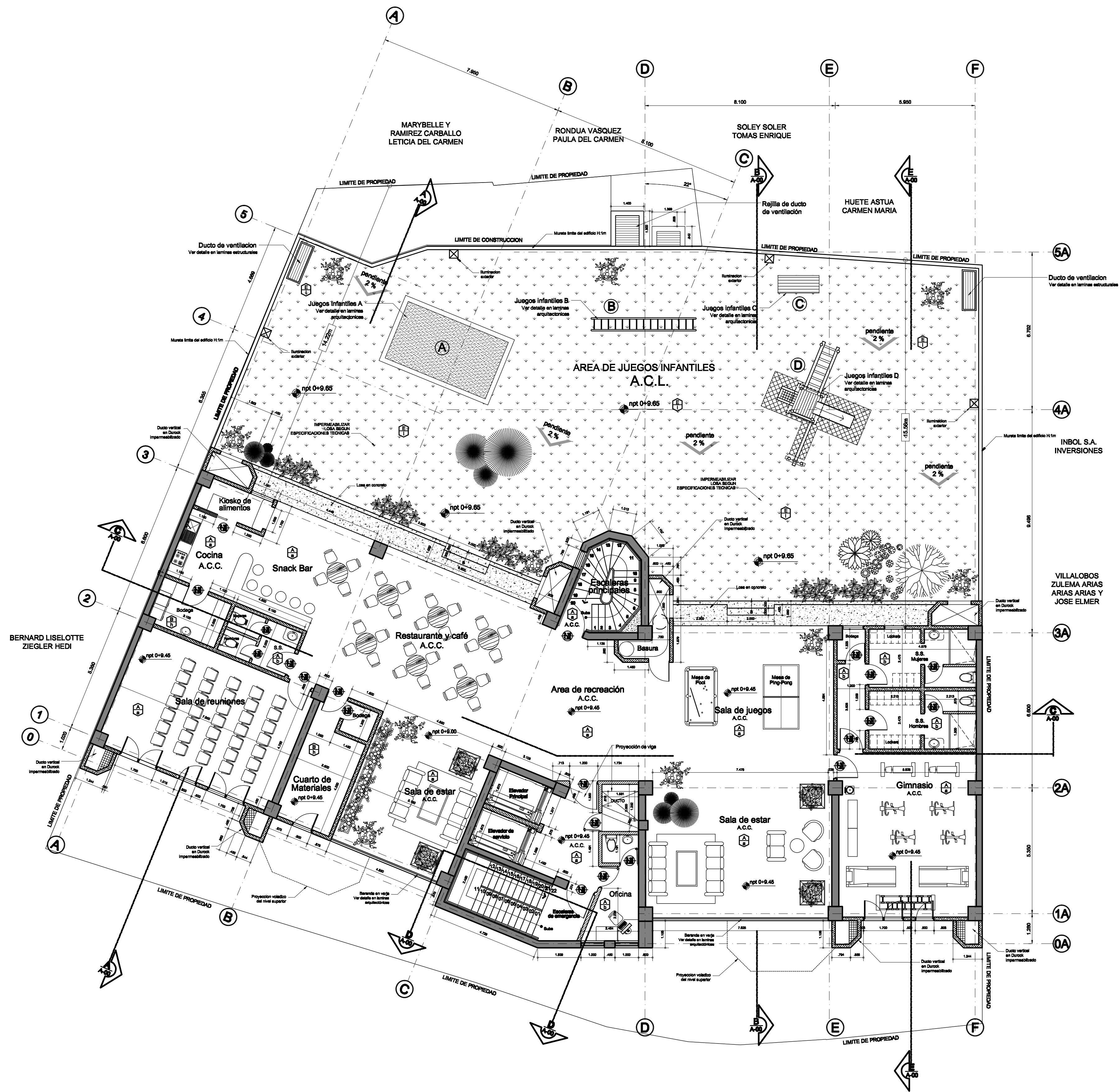
PLANTA DE DISTRIBUCION ARQUITECTONICA N I V E L 1 Nivel 0+9.45m ESCALA 1:75
