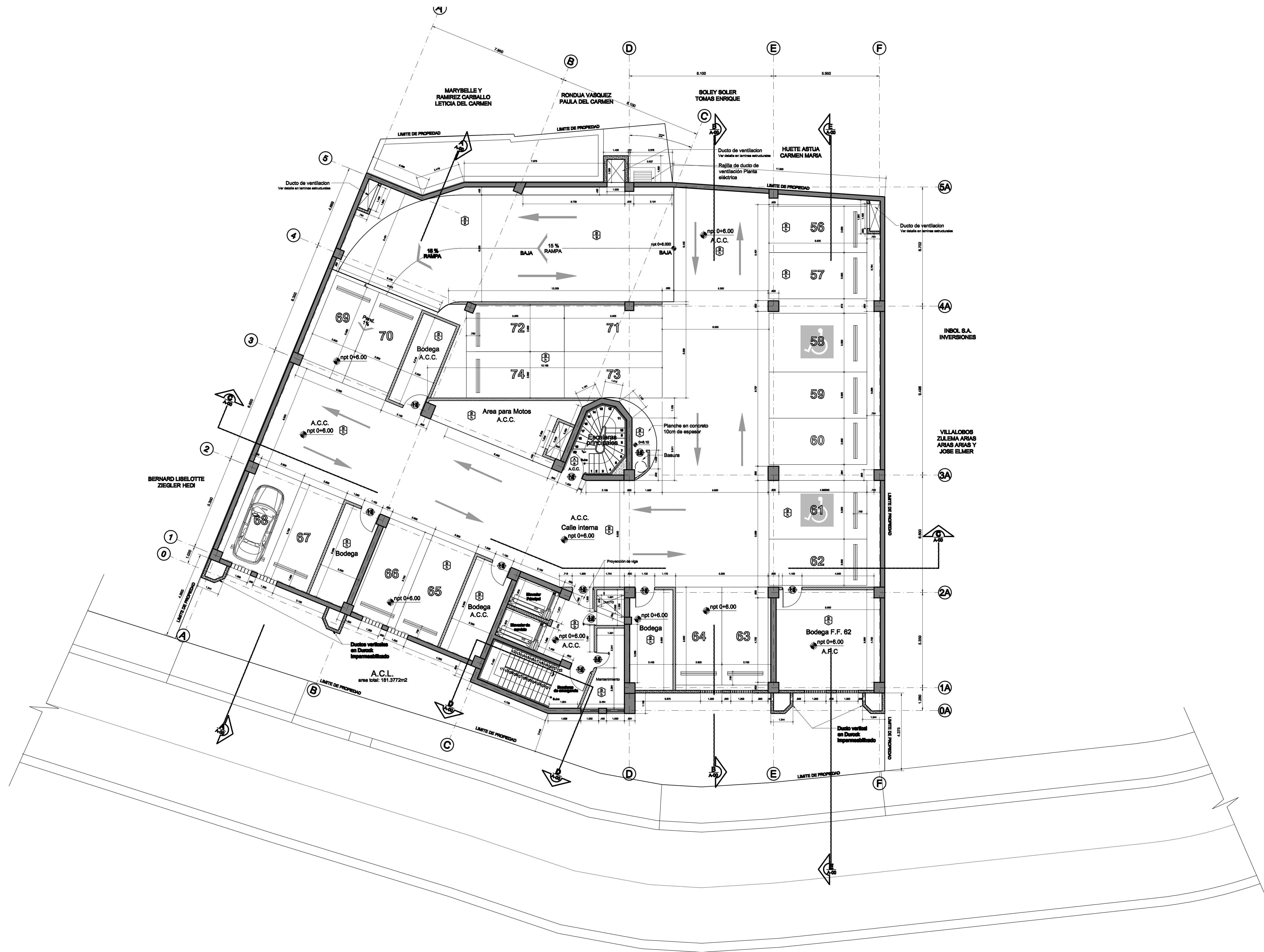
PLANTA DE DISTRIBUCION ARQUITECTONICA N I V E L Parqueo P1 Nivel 0+6.00m ESCALA 1: 75
