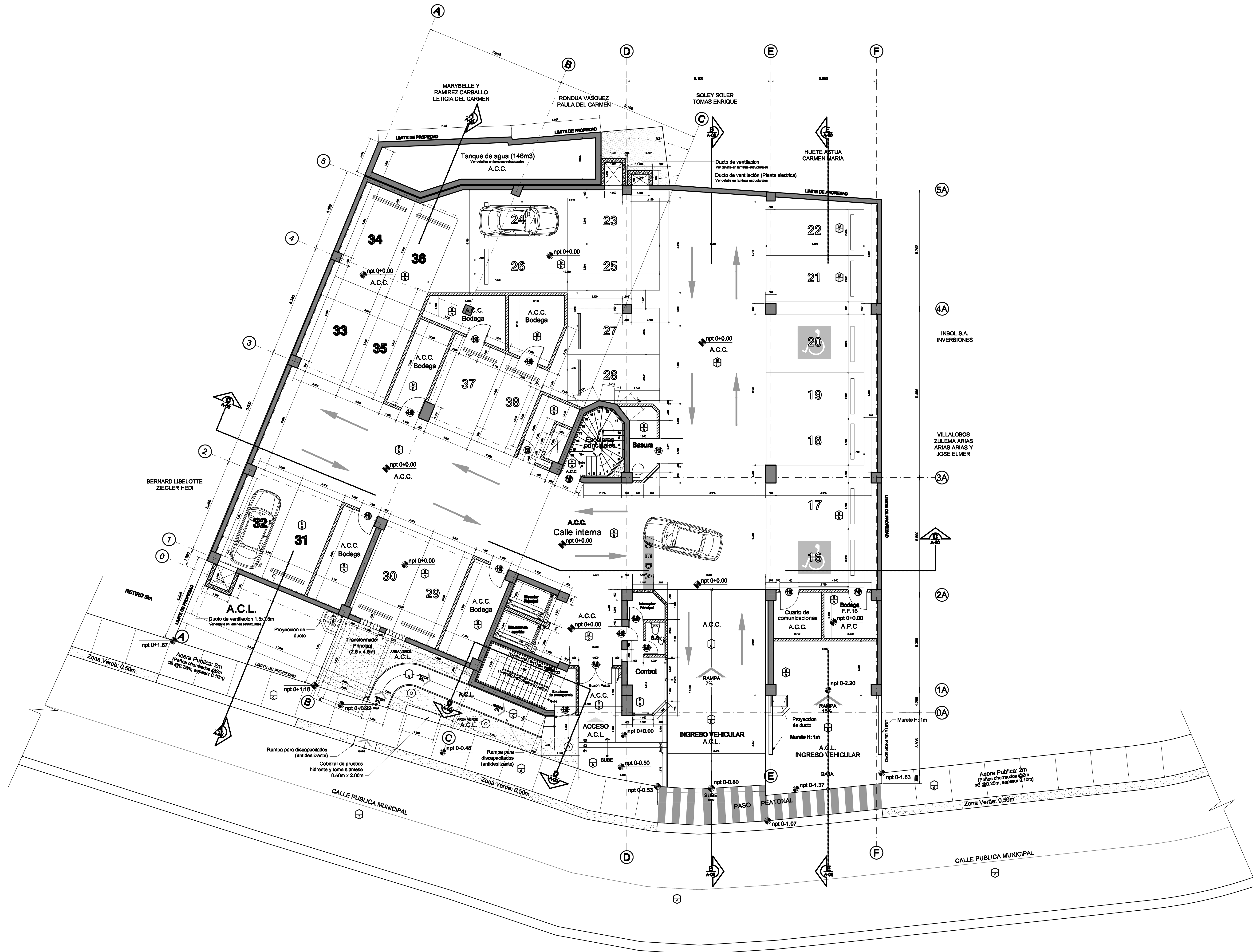
PLANTA DE DISTRIBUCION ARQUITECTONICA N I V E L Parqueo P3 Nivel 0+0.00m ESCALA 1: 75
