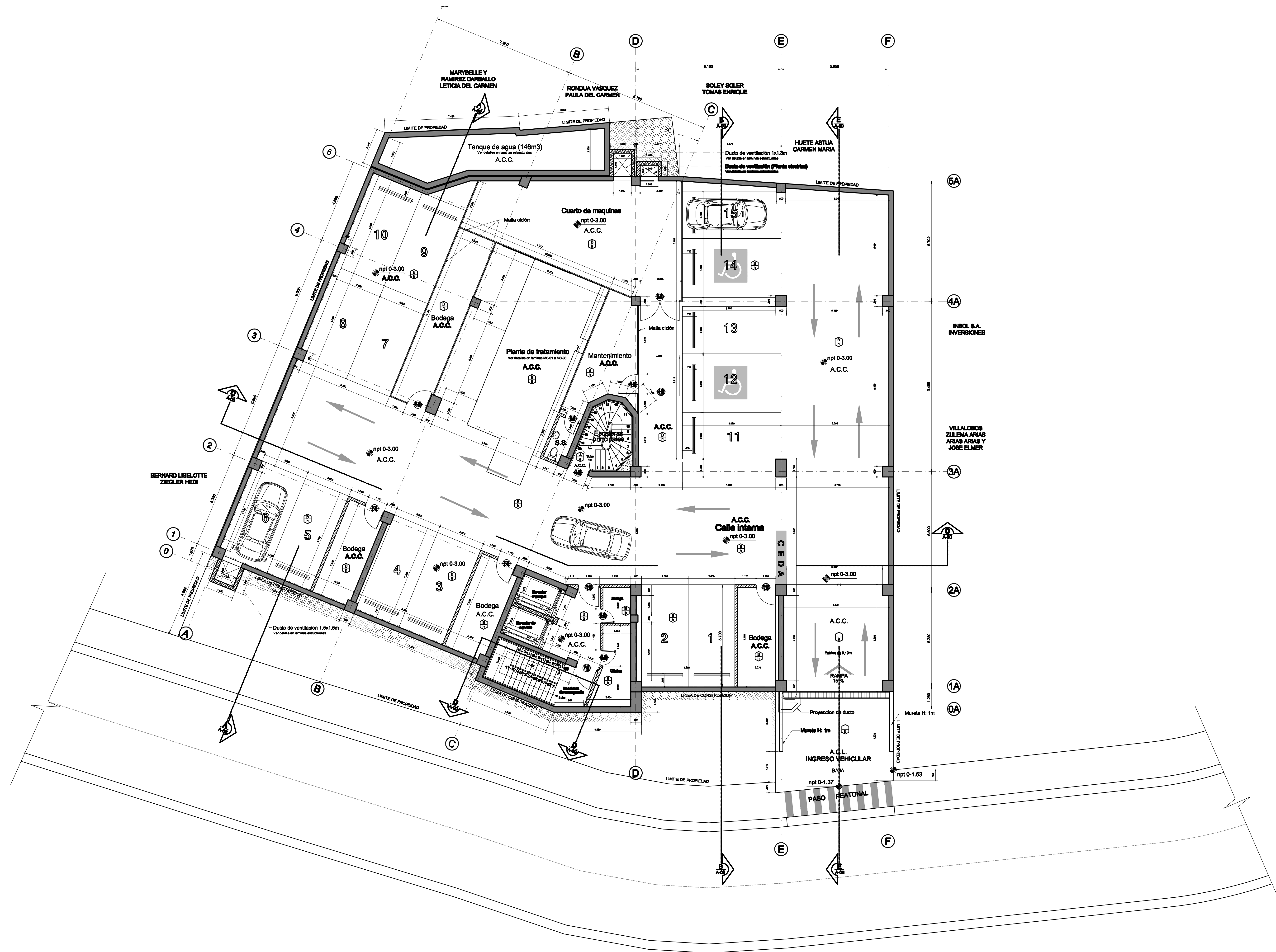
PLANTA DE DISTRIBUCION ARQUITECTONICA N I V E L Parqueo P4 Nivel 0-3.00m ESCALA 1: 75
